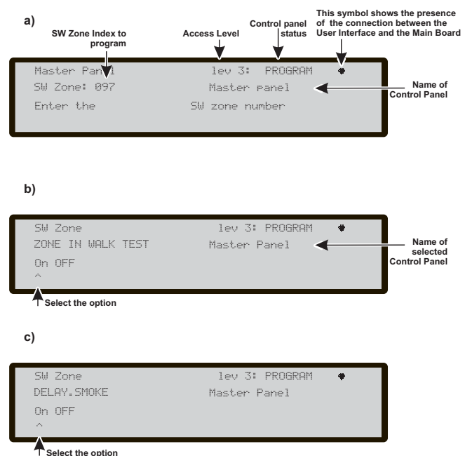
Figura 42 Pantalla Opción de programación retraso de activación de fumadores
