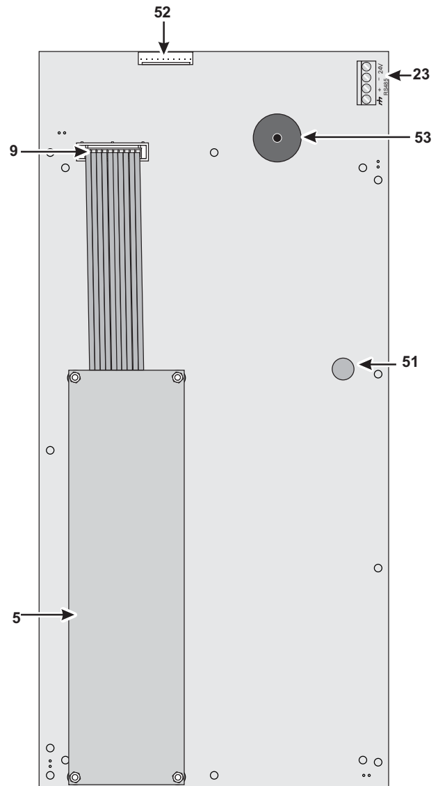
Figura 6 Identificación de las partes: Tarjeta LCD
