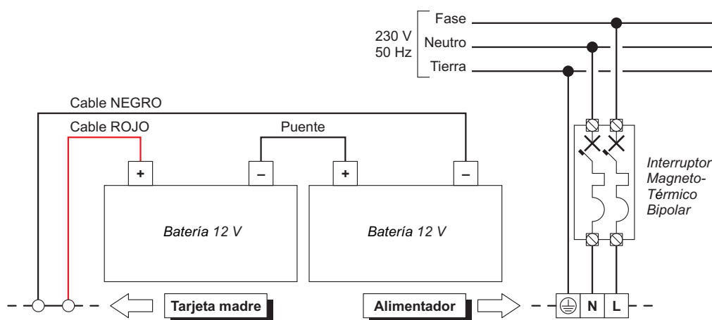
Figura 15 Conexión de alimentación
