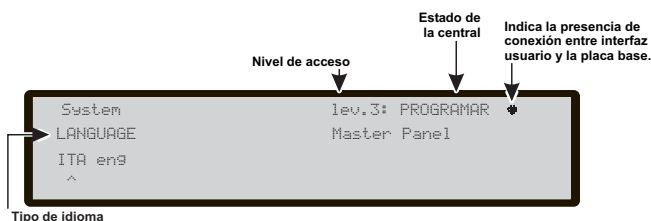
Figura 49 Pantalla para seleccionar el idioma del sistema: ITA-ENG
