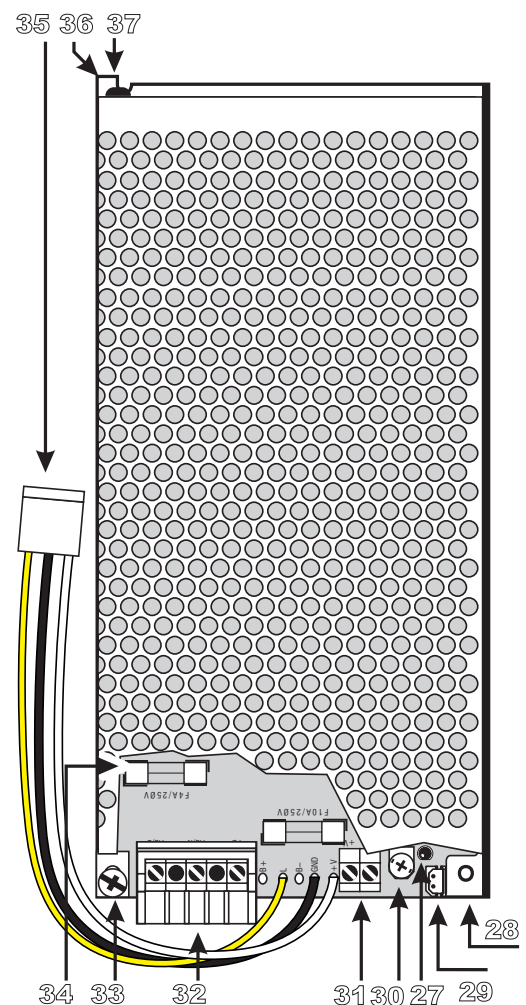
Figura 5 Alimentador BAQ140T24
