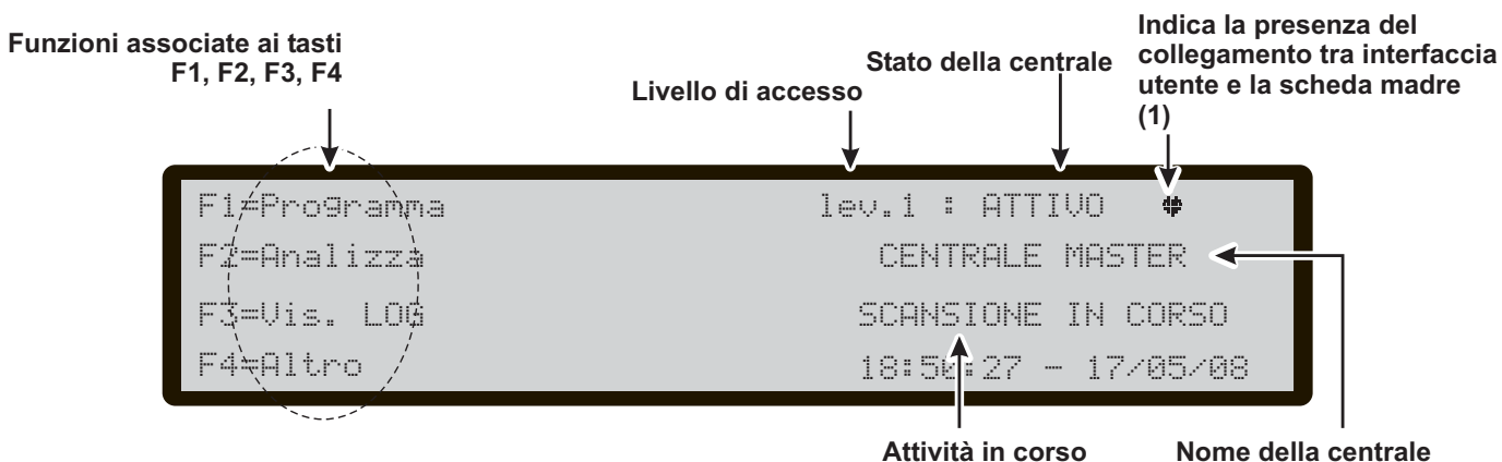
Figura 1 Schermata: STATO di RIPOSO-Accesso alla gestione della centrale; (1)- nel caso si tratti del Display di un Repeater , alternativamente al simbolo che indica la presenza del collegamento tra l'interfaccia e la scheda madre verrà mostrato l'indirizzo del repeater stesso.
